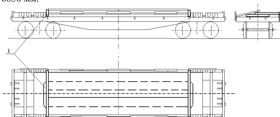
Рисунок 181 1 – балка упорная
